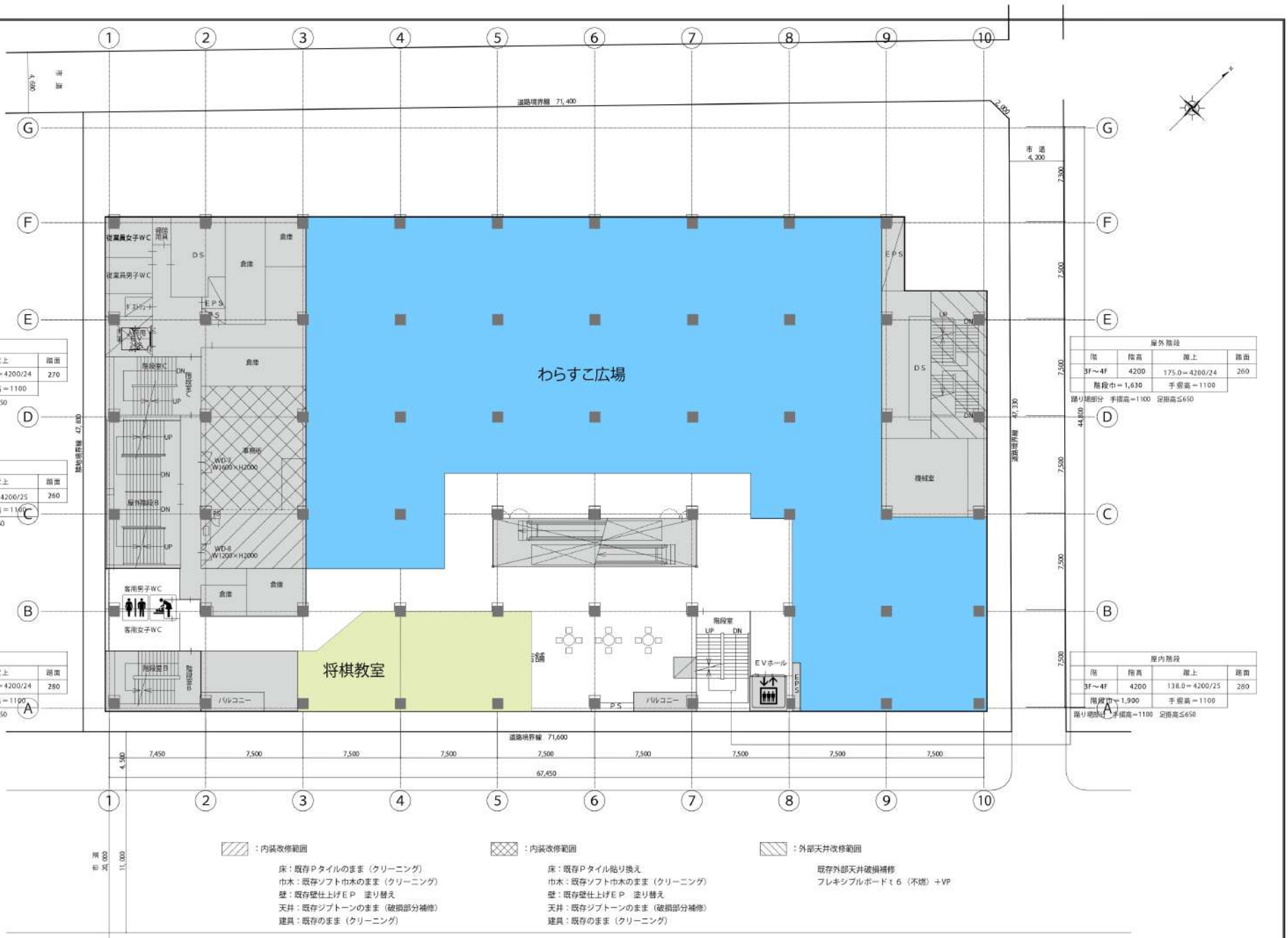
4階 平面図 1/200 ×100% (A2) ×71% (A3)
