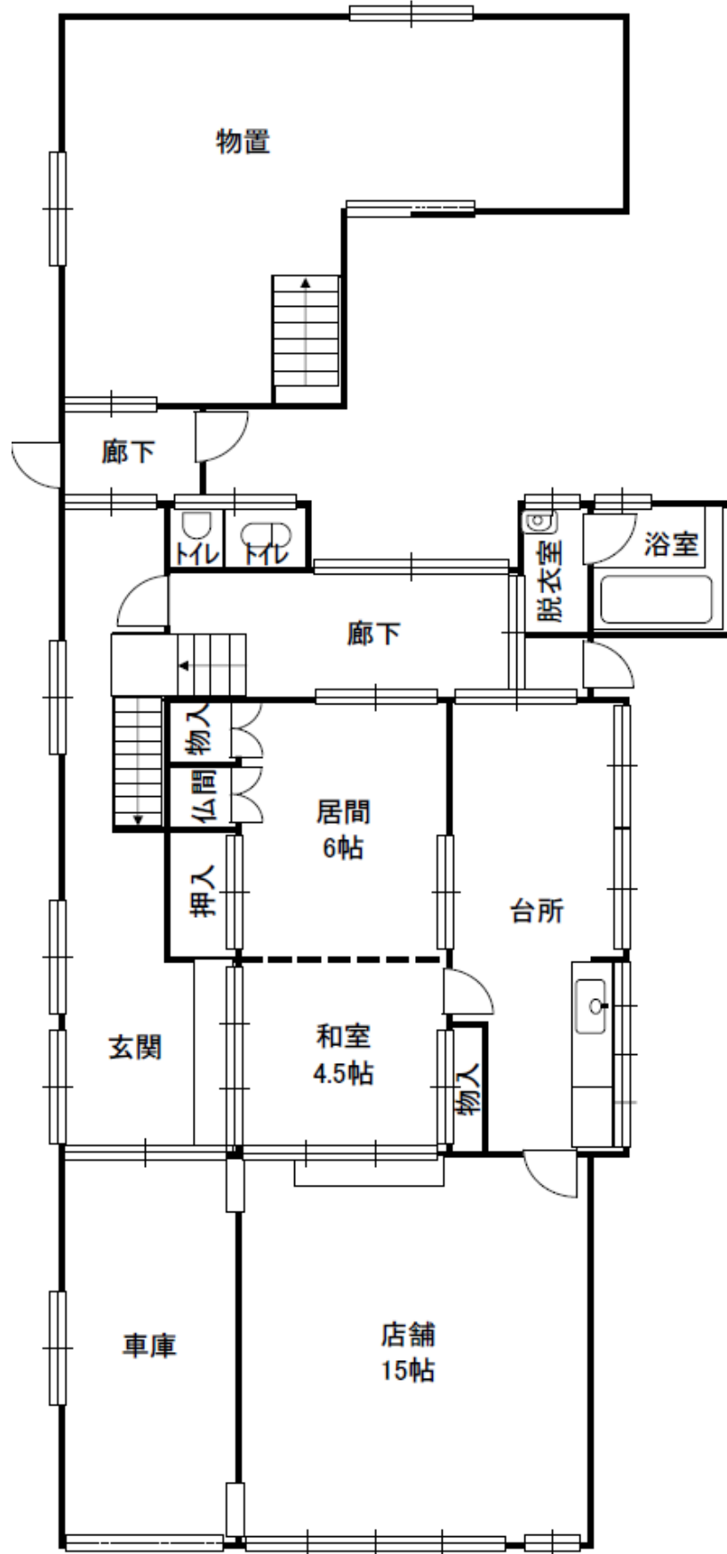
1階間取り
