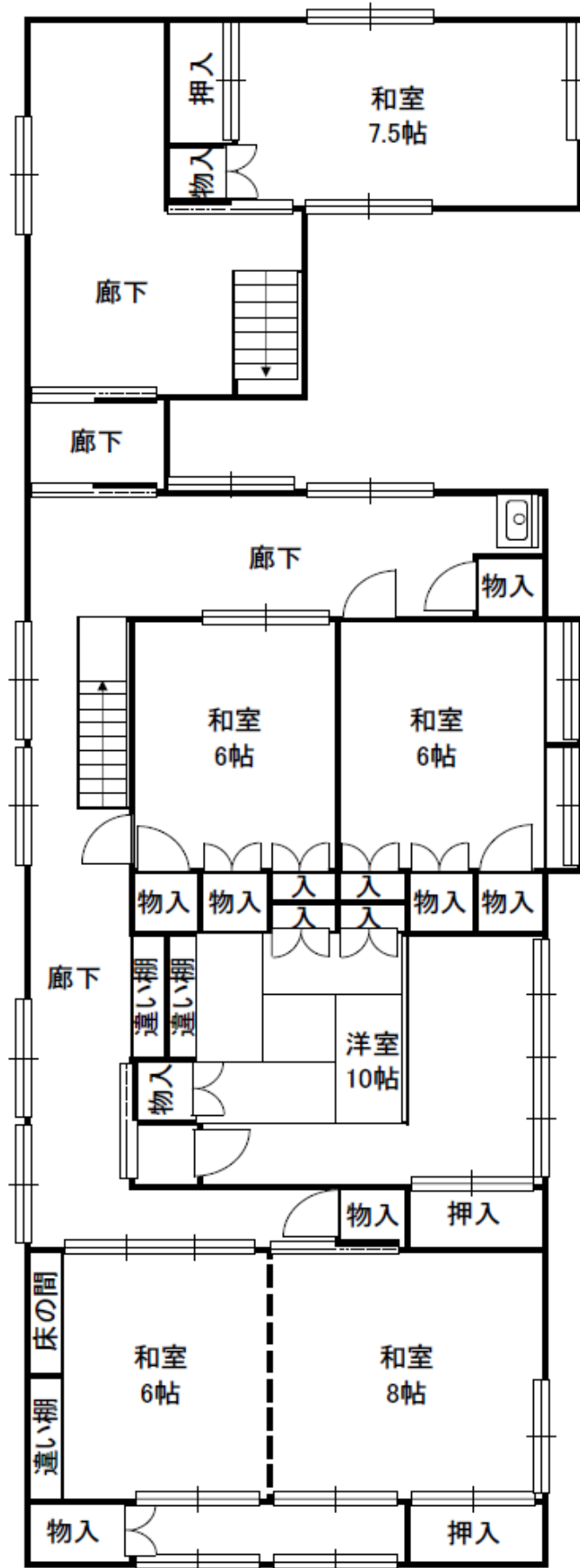
2階間取り
