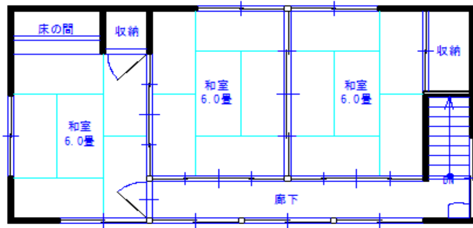
二階間取図
