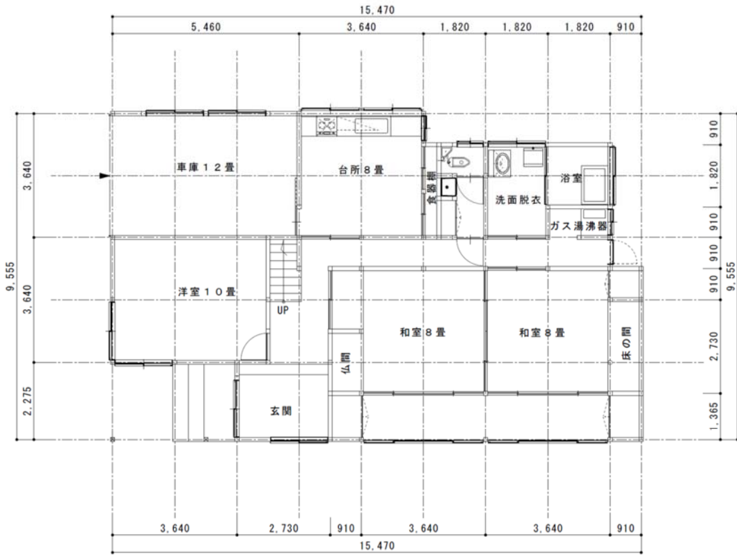
2階平面図
