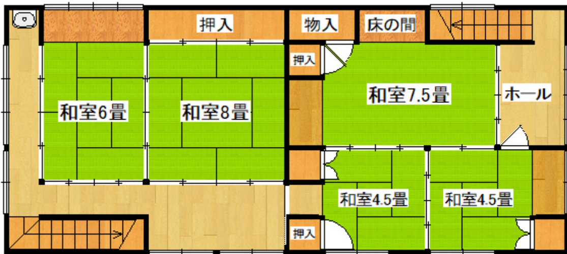
2階平面図
