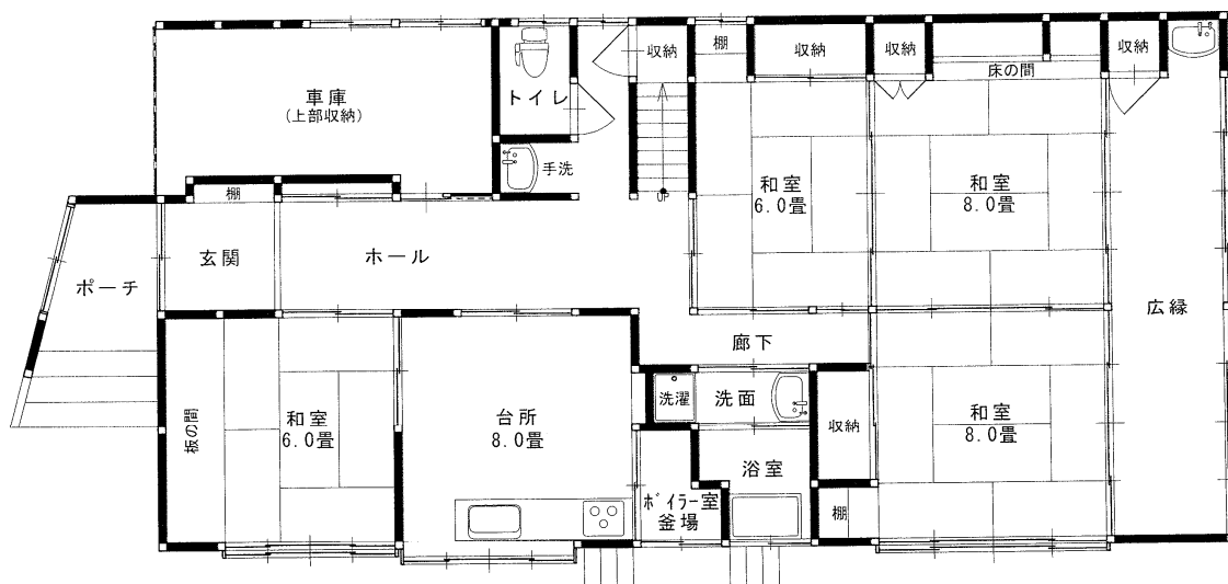
一階平面図 S = 1 / 100
