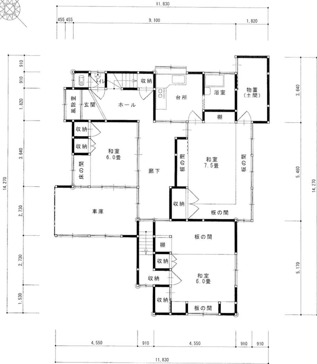
一階平面図 S = 1/100
