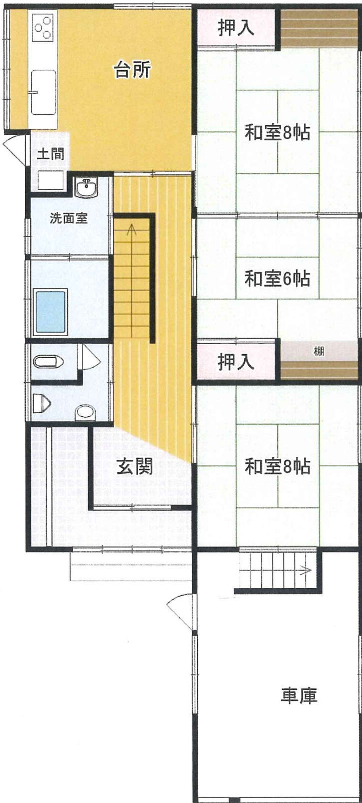
1階平面図
