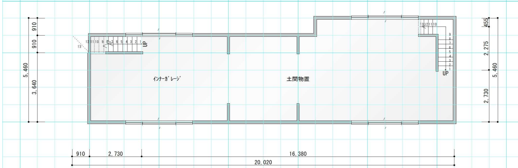
2F 平面図
