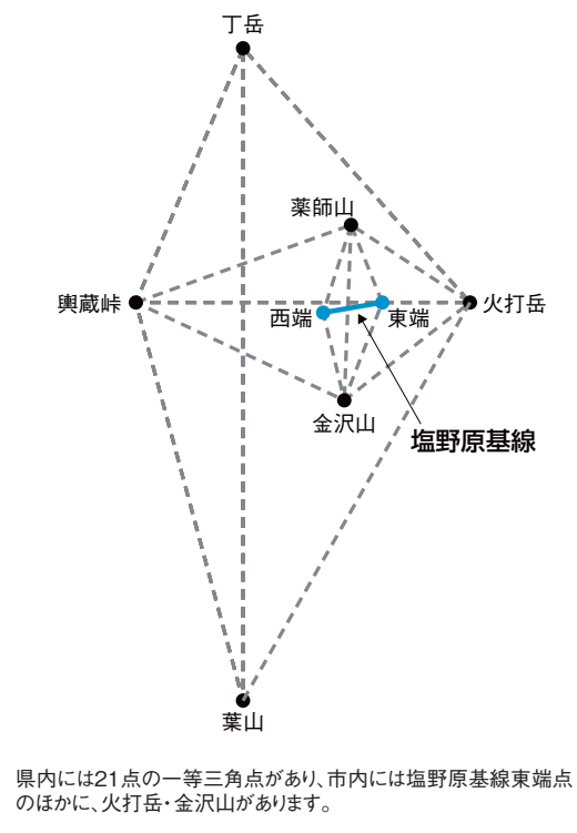
図2 塩野原基線と周辺の三角網形成
